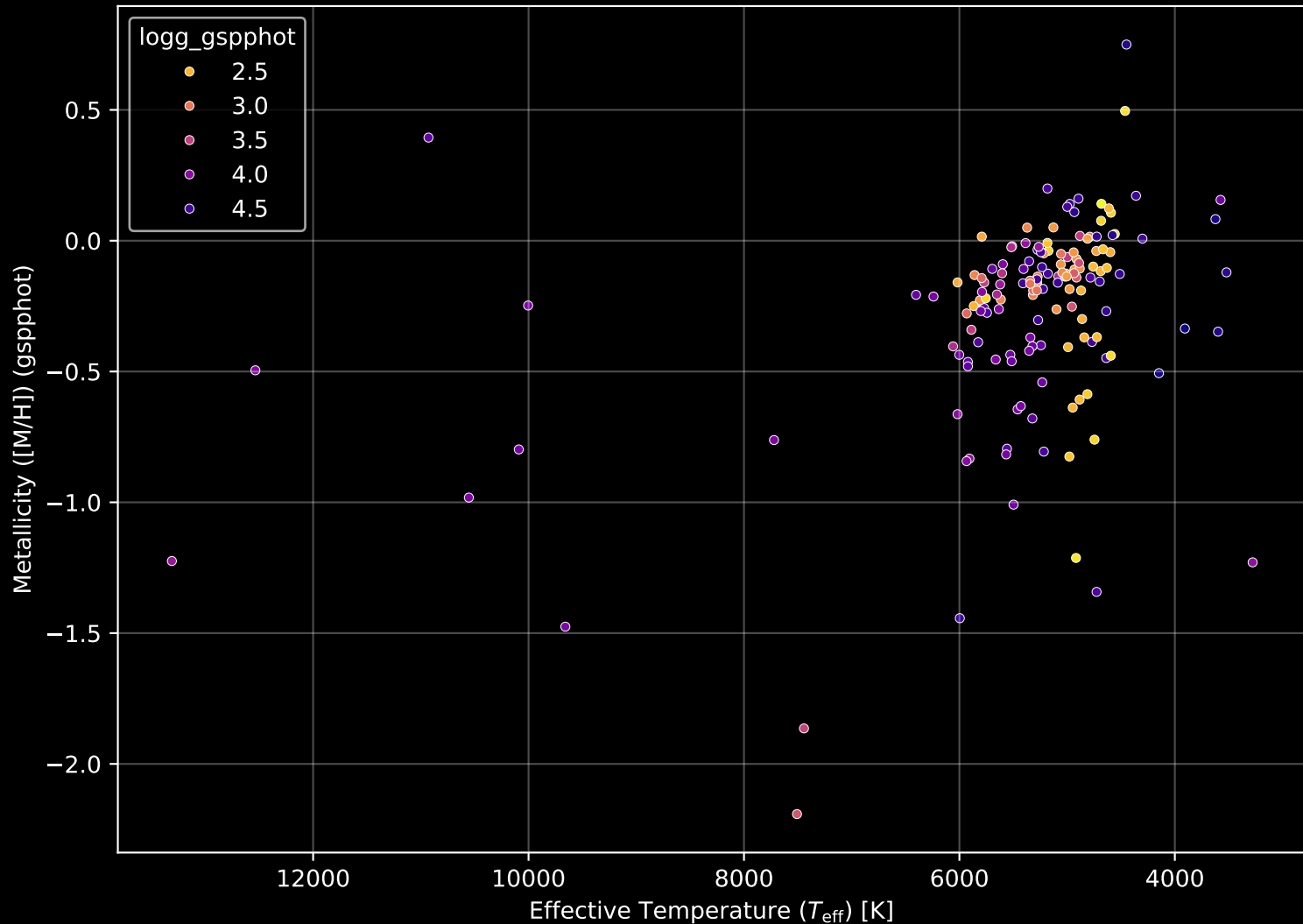
APOGEE DR17 Field: [K2_C13_171-20_btx] Stellar Population Parameters (n= 156)
